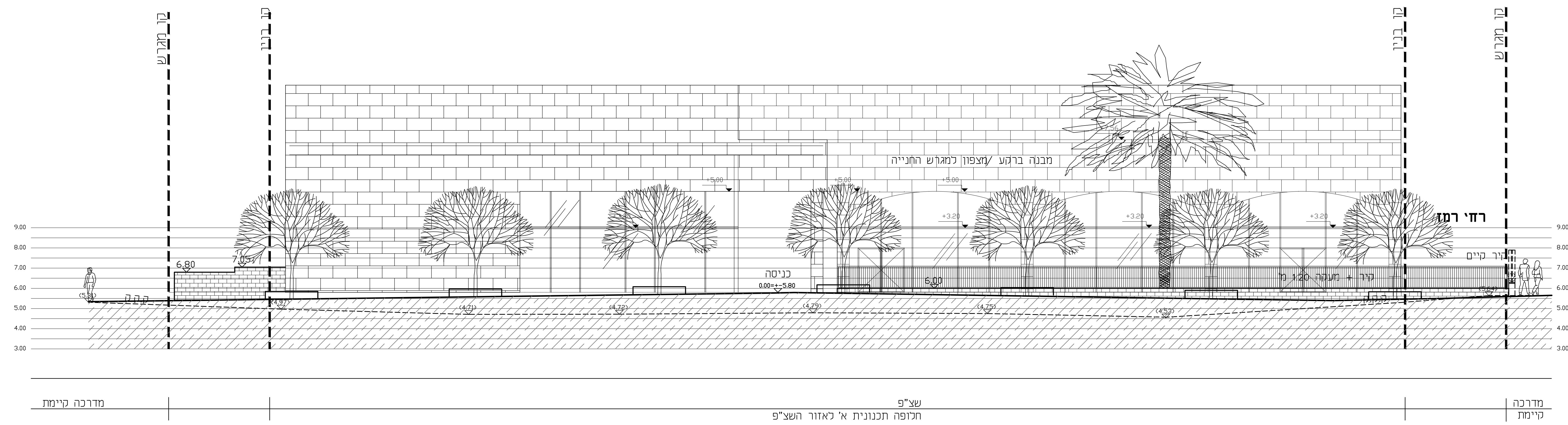
חזית דרומית
