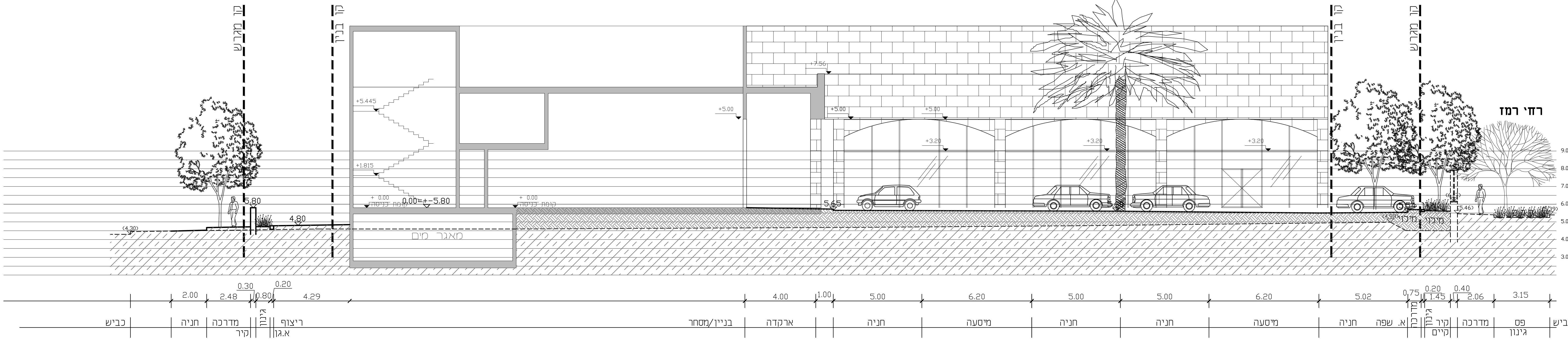
חזת ב-ב
