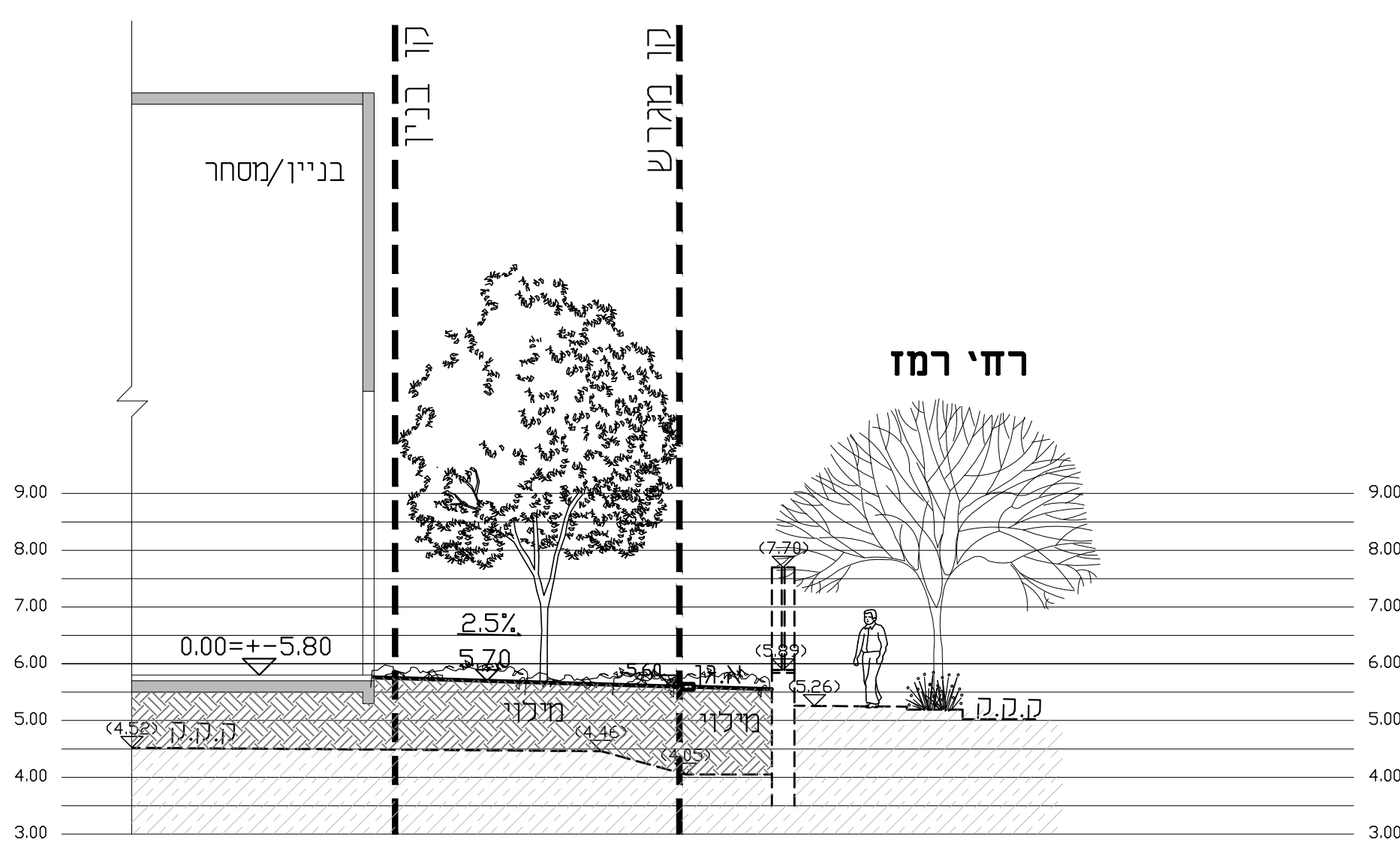
חזית מערבית
